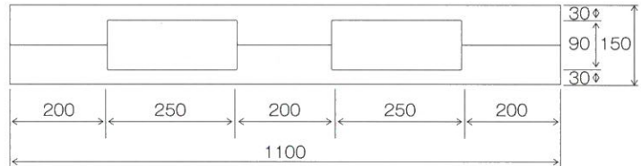
寸法図
